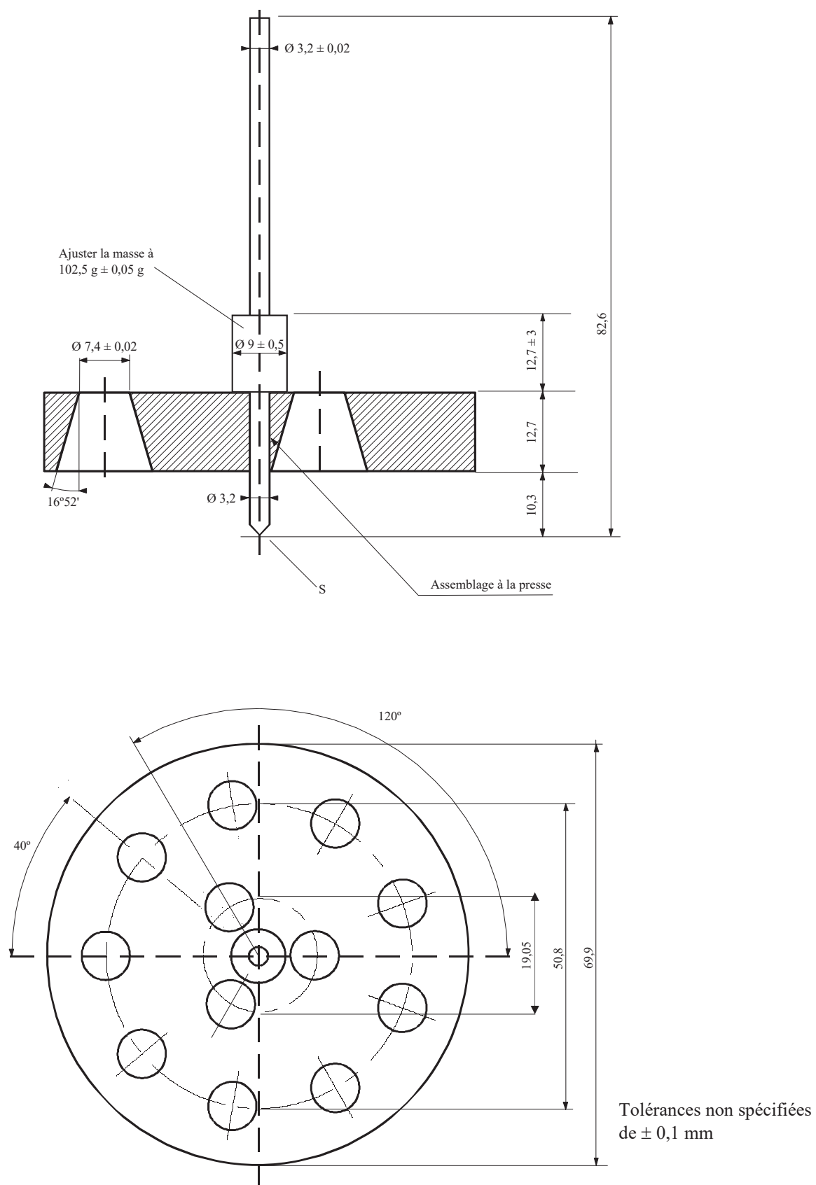
Figure 1 – Pénétromètre
